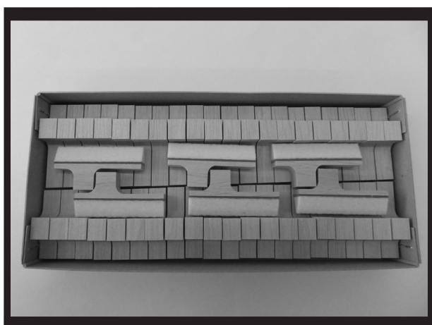
⑤ トレブルダンパーフェルトセット
