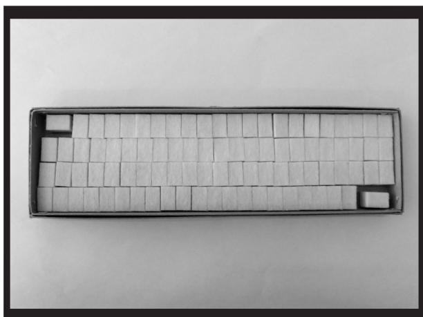
⑨ ハンマーシャンクストップフェルト
